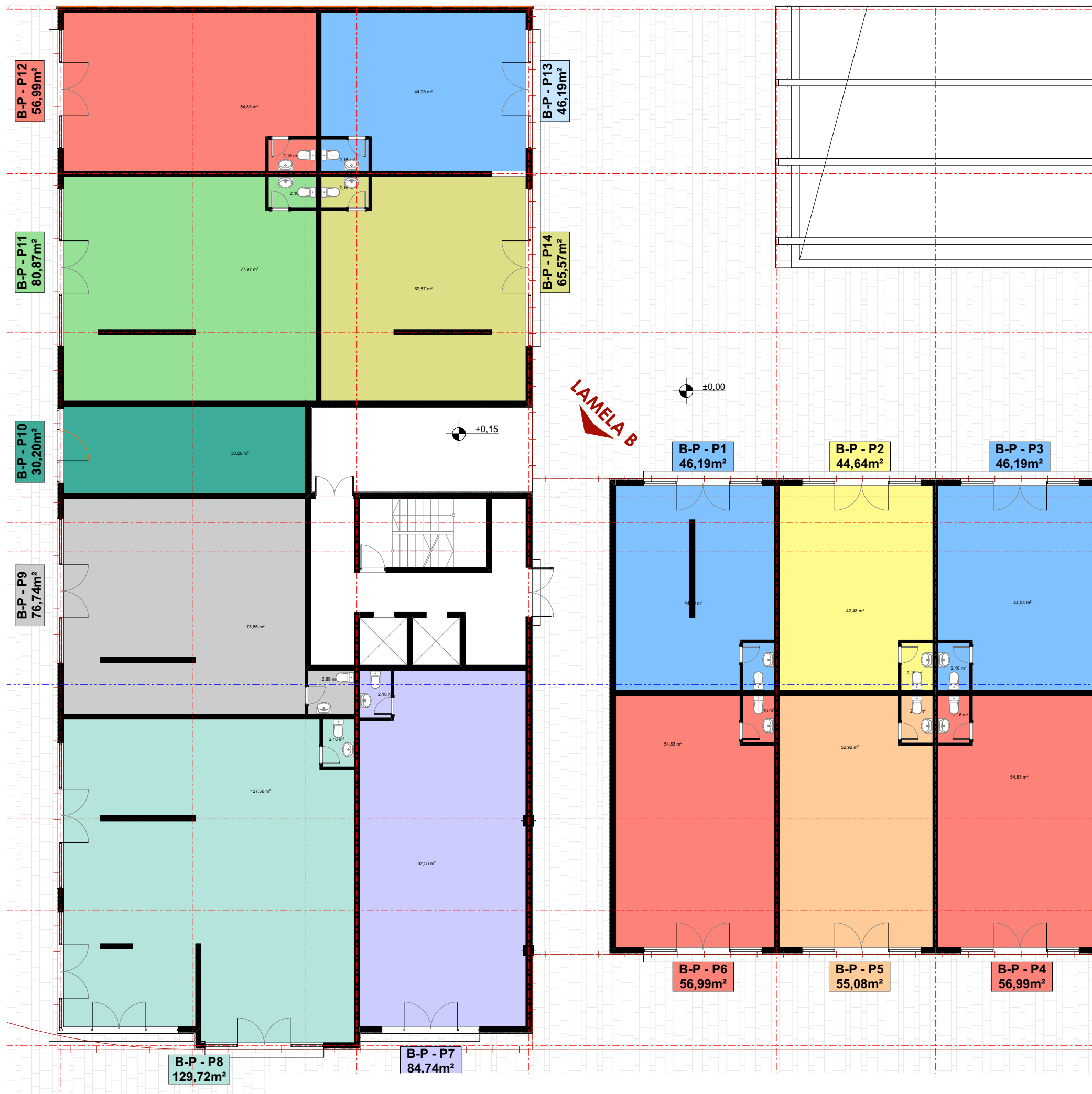
OSNOVA PRIZEMLJA R=1:150
