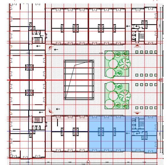
OSNOVA IV SPRATA R=1:100
