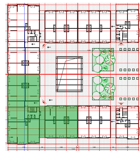
OSNOVA II SPRATA R=1:150
