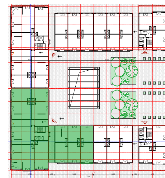
OSNOVA IX SPRATA R=1:100
