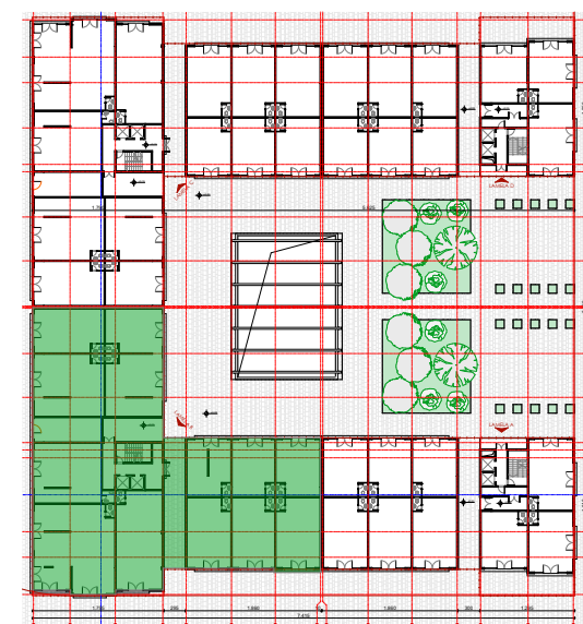
OSNOVA V SPRATA R=1:150
