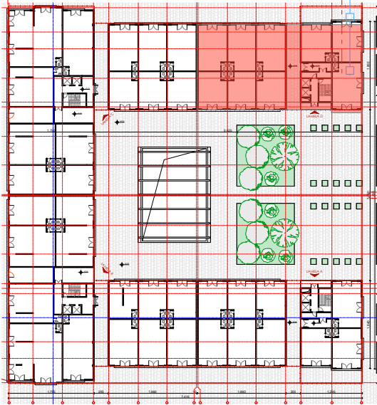
OSNOVA IV SPRATA R=1:100
