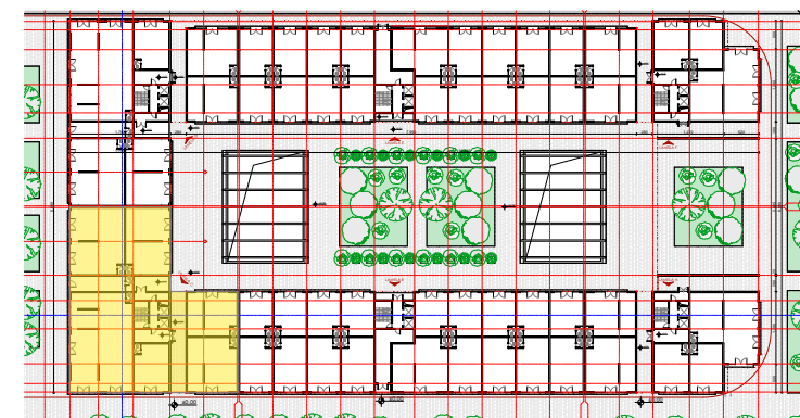
OSNOVA PRIZEMLJA R=1:150
