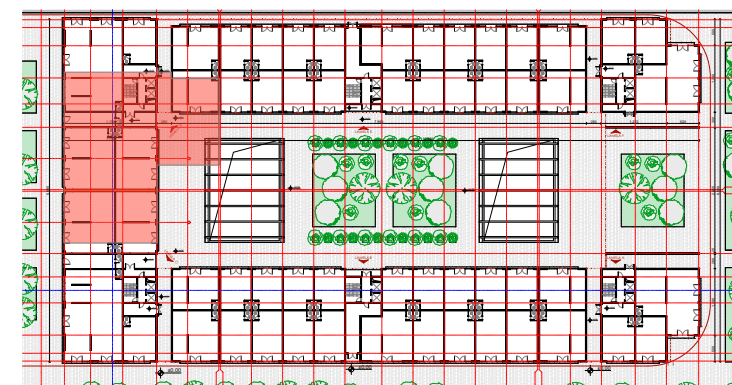
OSNOVA PRIZEMLJA R=1:150
